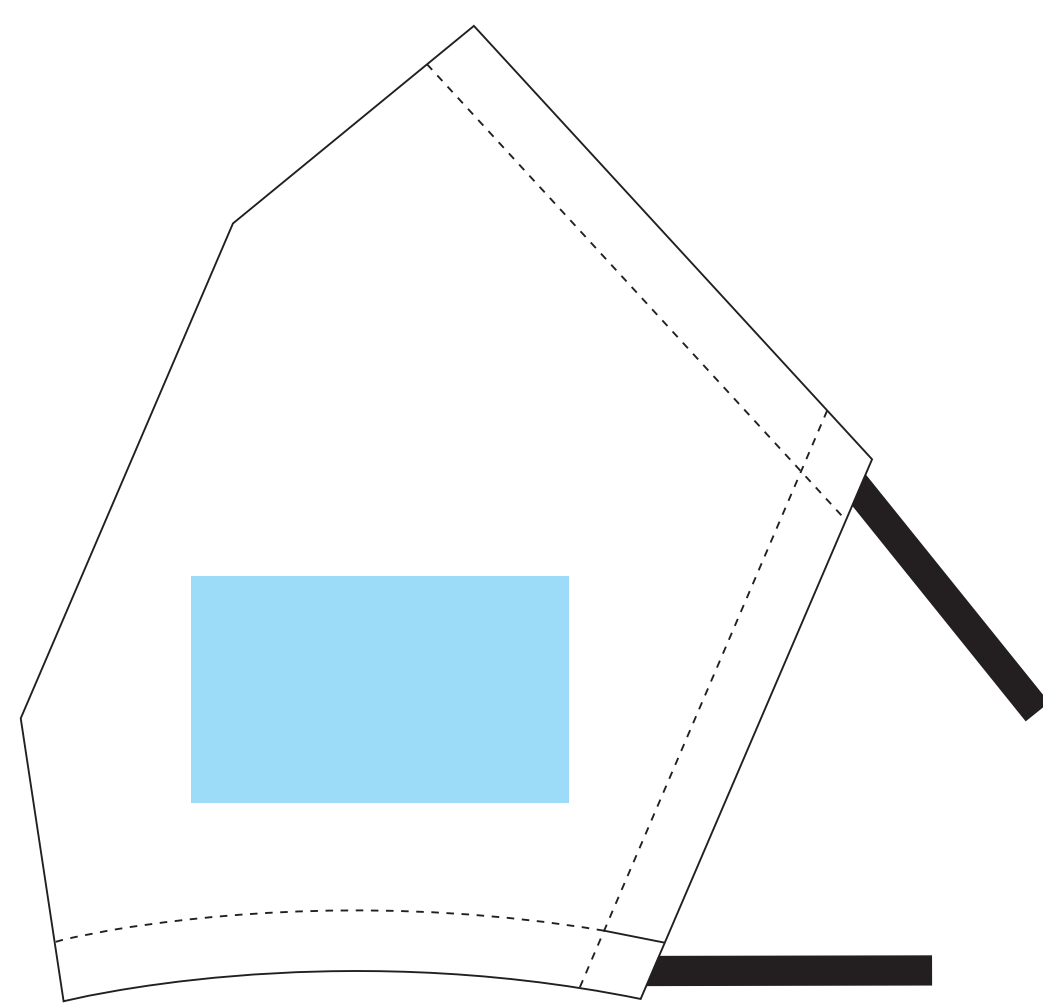
レイアウト A:W50×H30mm
