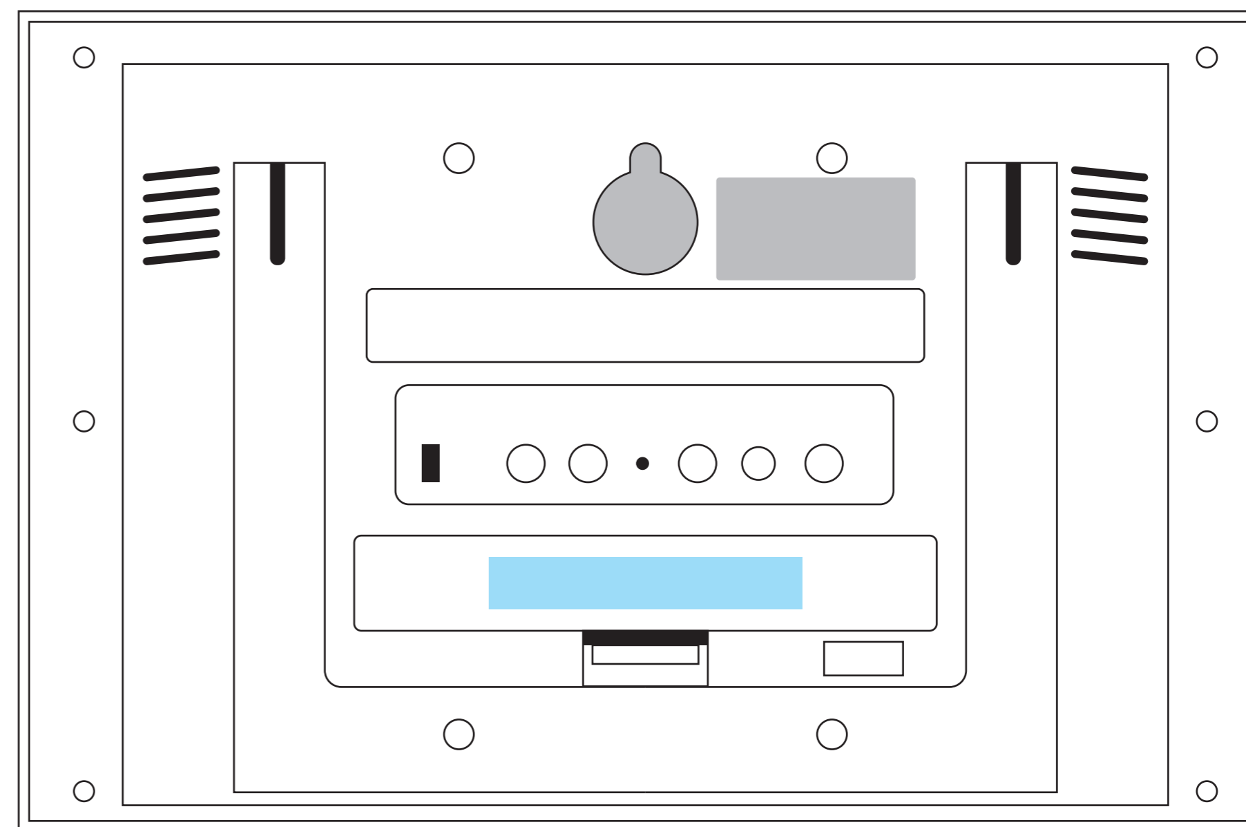
B(裏面電池蓋):W60×H10mm
